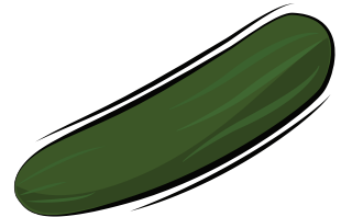
ἄσπερον
